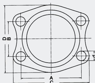
Brida según la norma SAE
