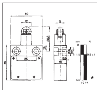
Membrane toggle roller lever 07-2951-..30/18
