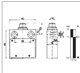
Roller plunger 07-2951-..30/09
